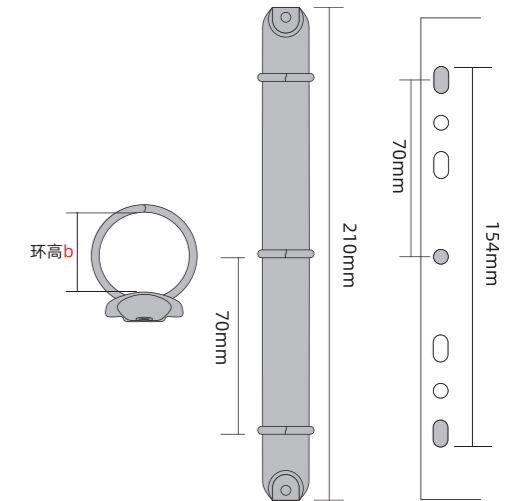
O形孔图: 铁夹图: 适用卡页孔位图:
