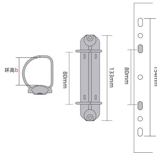
D形孔图: 铁夹图: 适用卡页孔位图:
