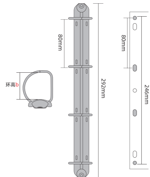
D形孔图: 铁夹图: 适用卡页孔位图:
