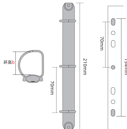
D形孔图: 铁夹图: 适用卡页孔位图:
