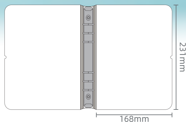
卡册内里结构图：
