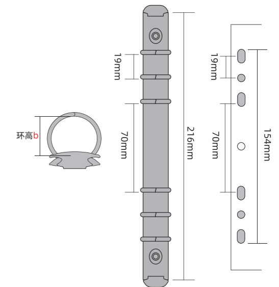
O形孔图: 铁夹图: 适用卡页孔位图:
